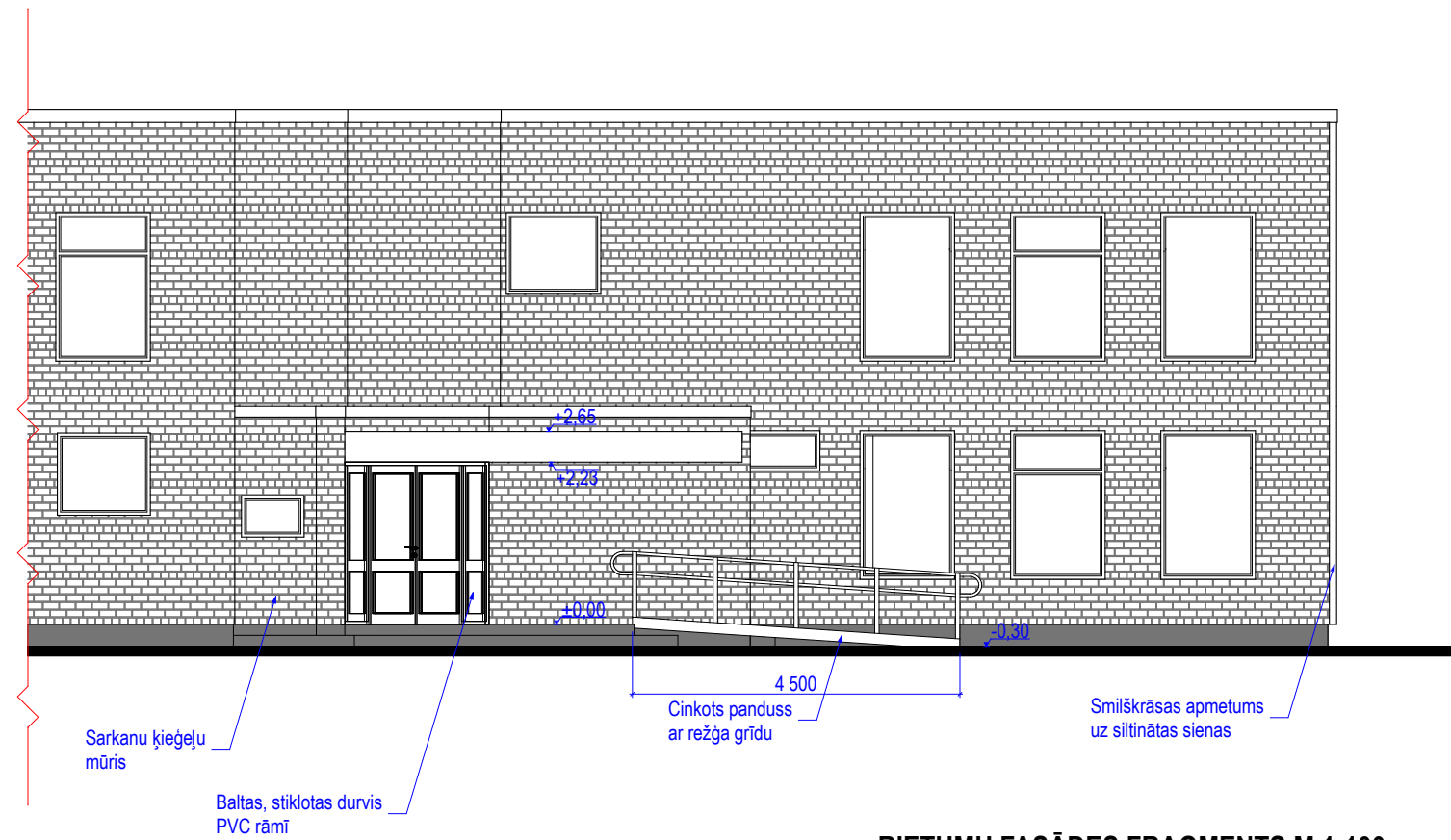
RIETUMU FASĀDES FRAGMENTS M 1:100
